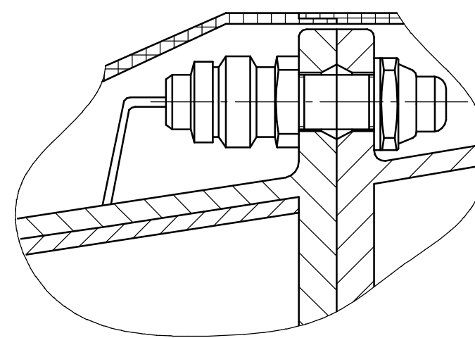
А (увеличено)
