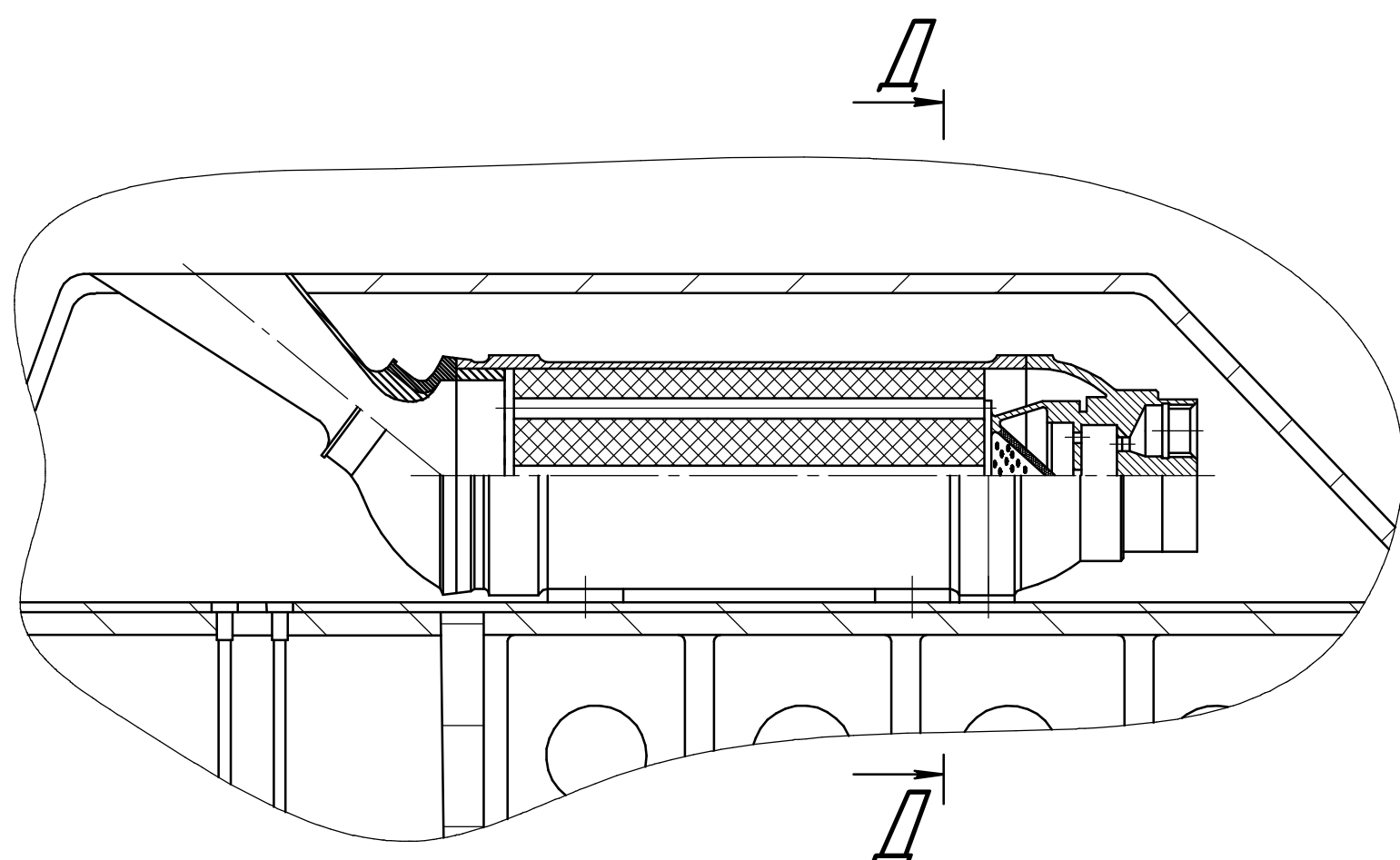
Г (увеличено)
